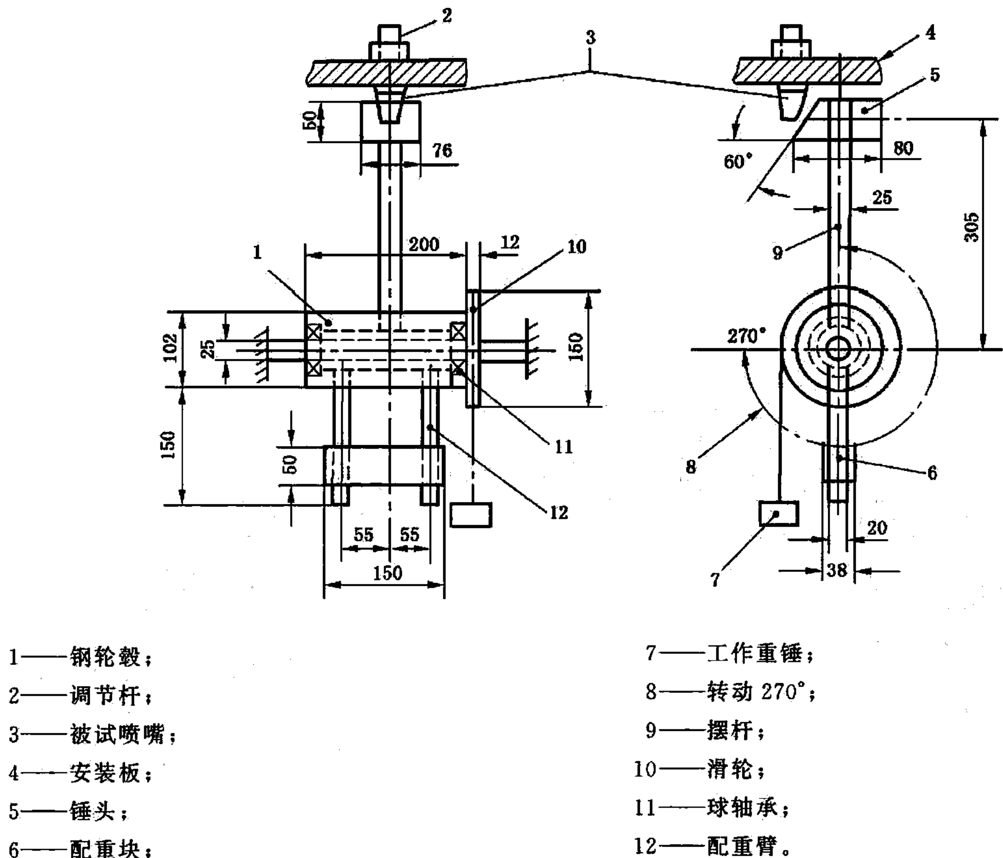
图 10 喷嘴耐冲击试验装置
